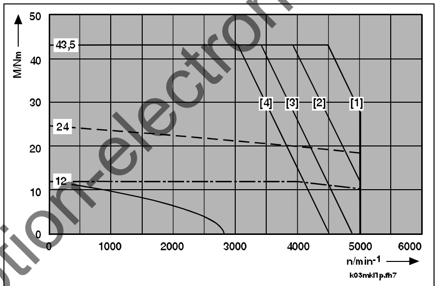
Fig. 8-8: Caractéristiques de vitesse de rotation – couple MKD090B-058
